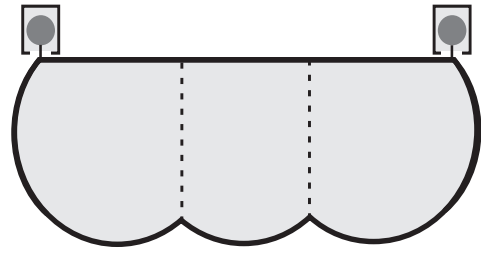
多半圆形组合式&大风量矩形织物风管示意图
