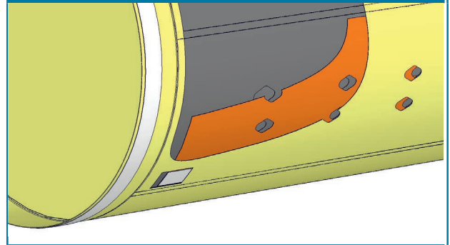
调节孔的部分由三层面料组成
